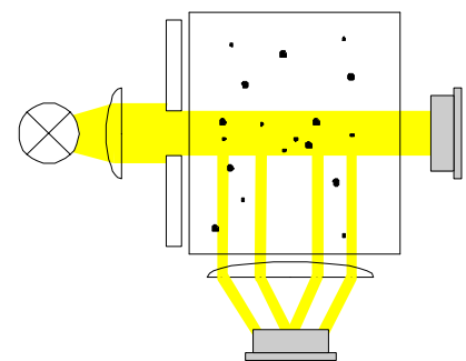
Système de mesure de la turbidité à 90° et double faisceaux
